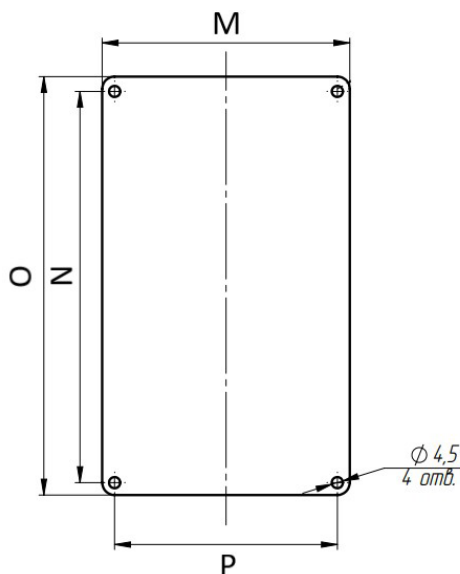
Рисунок 2.7–3. Чертеж нижней крышки преобразователя частоты J1-J12
