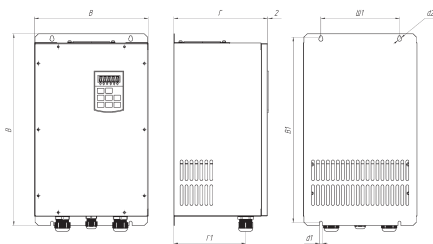
Рис. 2.7 Габаритные и установочные размеры устройств серии LCI в корпусе IP54
