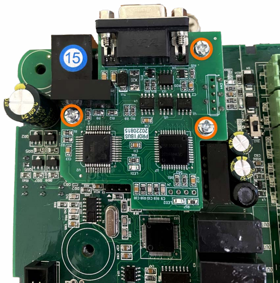
Рисунок 11 – Крепежные винты платы расширения SNI-DP-S
