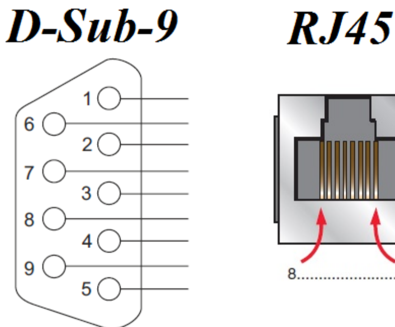
Рисунок 1 – Распиновка D-Sub-9-RJ45
