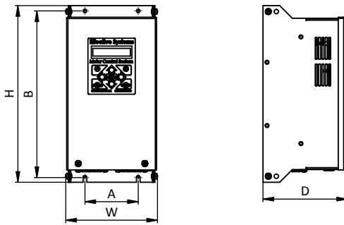
Рис. 2.1 Размеры контроллера 5,5 - 11 кВт
