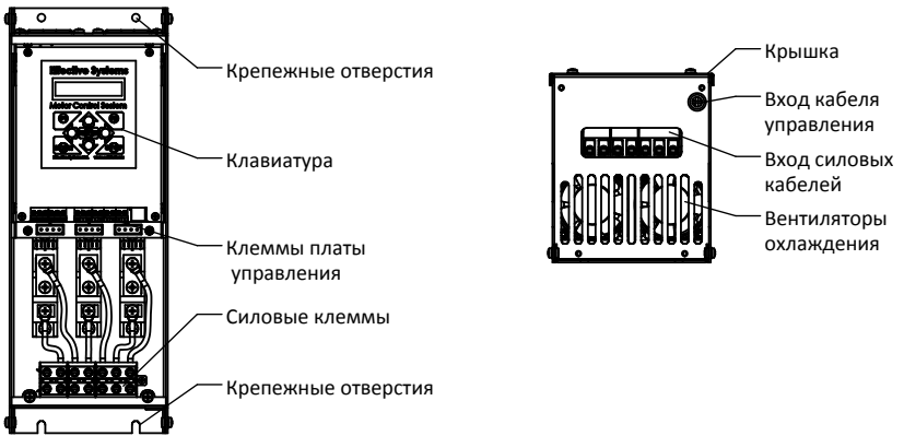
Рис. 1.2 Составные части контроллера номинальной мощностью 15 - 22 кВт
