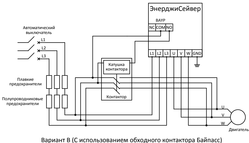
Рис. 7.1 Вариант подключения контроллера ЭнерджиСейвер без обходного контактора.
