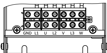
Силовые клеммы контроллеров мощностью 15-37 кВт
