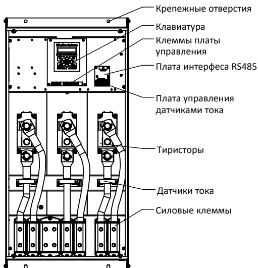
Рис. 1.7 Составные части контроллера номинальной мощностью 200 кВт
