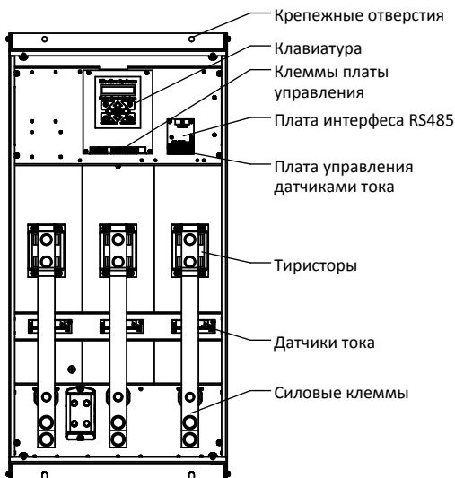
Рис. 1.8 Составные части контроллера номинальной мощностью 225 - 250 кВт
