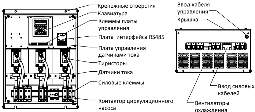
Рис. 1.5 Составные части контроллера номинальной мощностью 75 - 110 кВт
