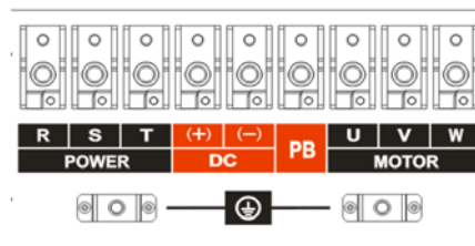
Рис. 3-14. Схема силовых клемм ПЧ мощностью 45~90 кВт
