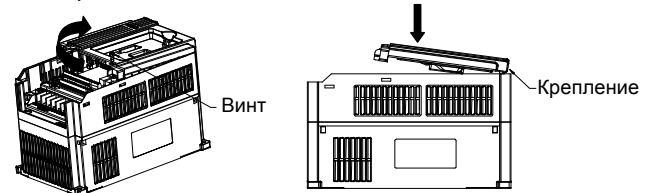
Рис. 3-7(ф). Демонтаж и монтаж кожуха
