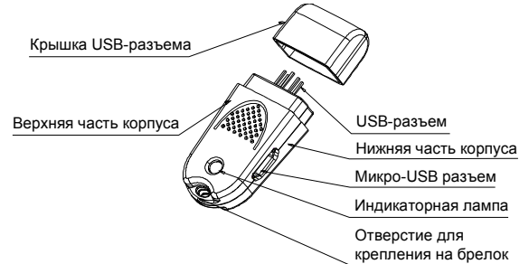
Рисунок В-1. Схема устройства модуля выгрузки и загрузки
