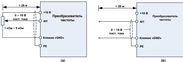
Рис. 3-16. Схема электропроводки клеммы аналогового входа
