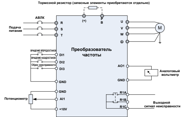
Рисунок 6. Схема подключения
