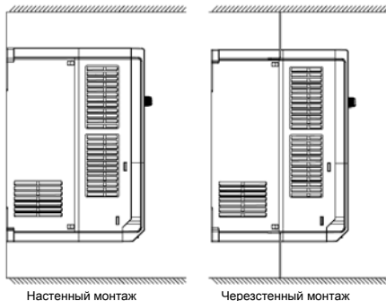
Настенный монтаж
