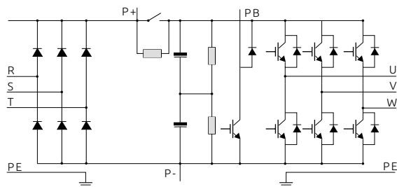
Рисунок 2-1. Схема силовой части(до 18,5 кВт (включительно))
