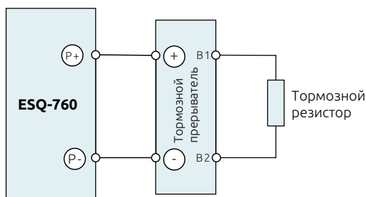
Рисунок 2-16. Подключение тормозного прерывателя.
