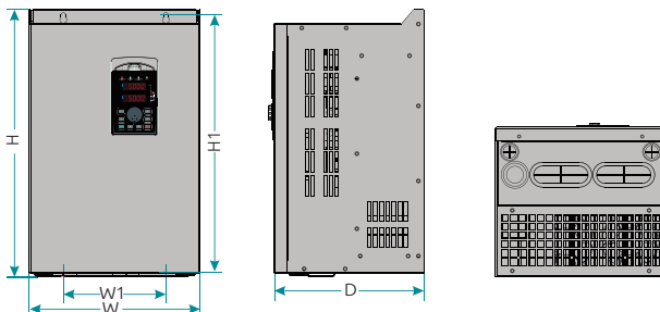
Рисунок 2-7. Установочные размеры ПЧ мощностью до 11-45 кВт
