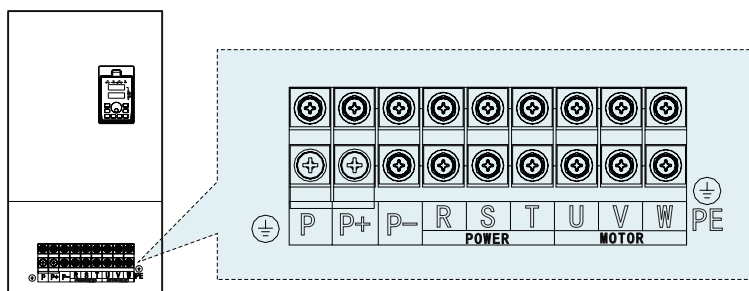
Рисунок 3-13. Схема силовых клемм ПЧ мощностью 55-110 кВт.
