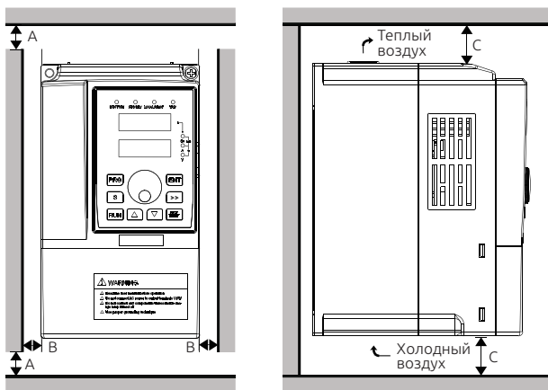
Рисунок 3-3. Установка одного преобразователя.
