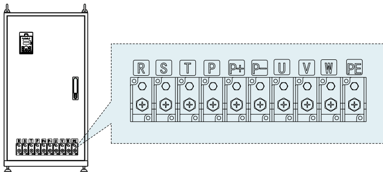
Рисунок 3-14. Схема силовых клемм ПЧ мощностью 132-185 кВт.
