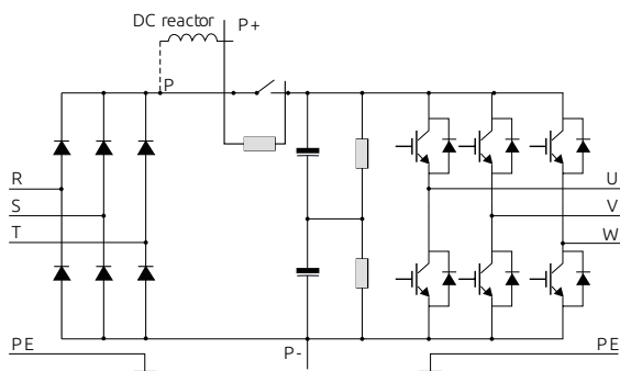
Рисунок 2-3. Схема силовой части(Больше 30кВт)
