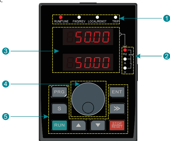
Рисунок 4-1. Внешний вид пульта управления.
