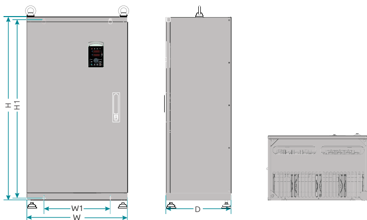
Рисунок 2-9. Установочные размеры ПЧ мощностью 132 - 185 кВт
