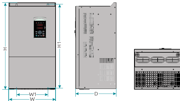
Рисунок 2-8. Установочные размеры ПЧ мощностью до 55 - 110 кВт
