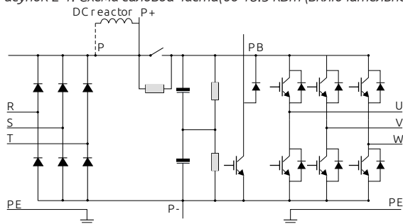
Рисунок 2-2. Схема силовой части(22кВт — 30кВт)
