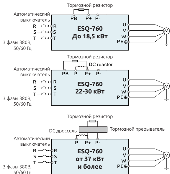
Рисунок 3-7. Основные схемы подключения.
