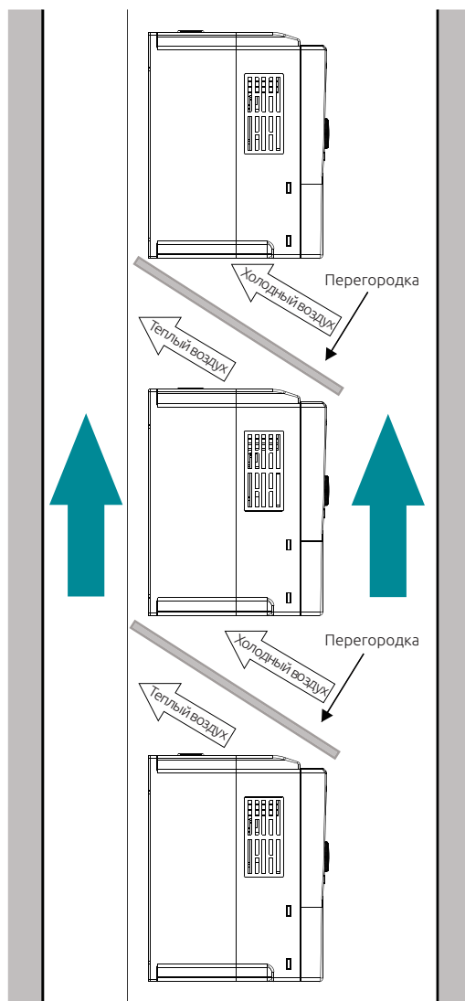
Рисунок 3-5. Вертикальная установка.
