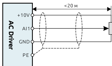
Рисунок 3-18. Схема подключения аналогового сигнала.
