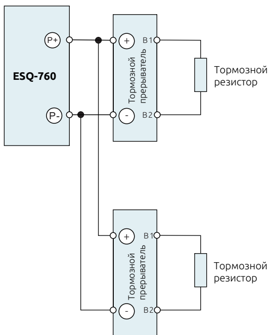
Рисунок 2-17. Параллельное подключение тормозных прерывателей
