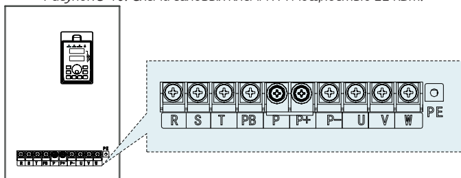
Рисунок 3-11. Схема силовых клемм ПЧ мощностью 30 кВт.
