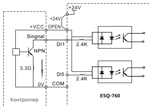
Рисунок 3-19. Подключение внешнего контроллера в режиме «Sink».
