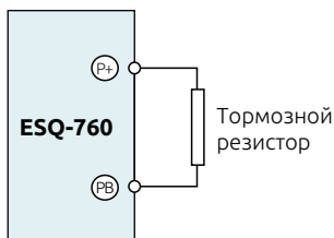
Рисунок 2-15. Подключение тормозного резистора к преобразователю мощностью до 22кВт
