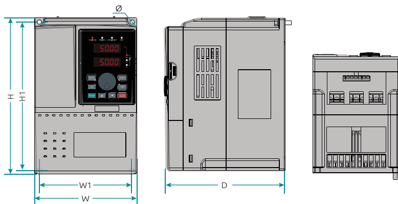
Рисунок 2-6. Установочные размеры ПЧ мощностью до 7,5 кВт включительно
