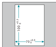
Рисунок 2-13. Размеры пульта без крепежного основания
