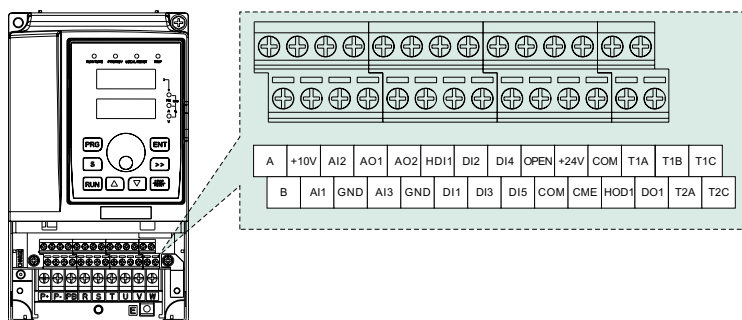
Рисунок 3-17. Клеммы управления.
