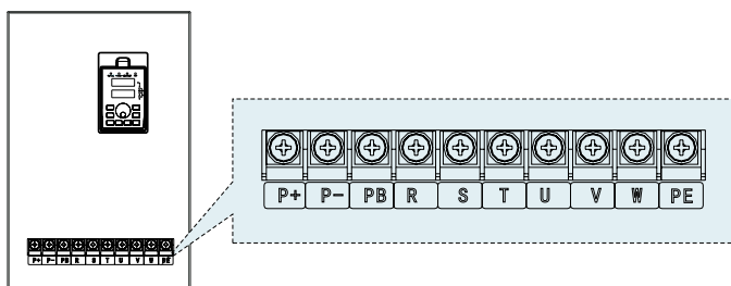
Рисунок 3-9. Схема силовых клемм ПЧ мощностью 11-18,5 кВт.
