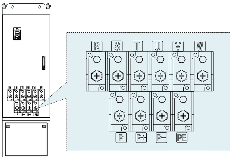
Рисунок 3-15. Схема силовых клемм ПЧ мощностью 200-500 кВт.
