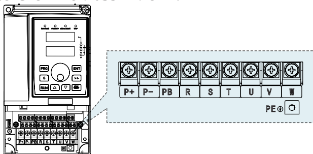
Рисунок 3-8. Схема силовых клемм ПЧ мощностью до 7,5 кВт.
