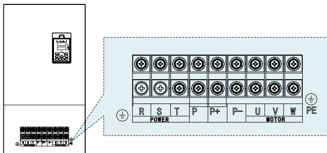
Рисунок 3-12. Схема силовых клемм ПЧ мощностью 37-45 кВт.
