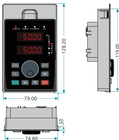
Рисунок 2-11. Установочные размеры выносного пульта управления
