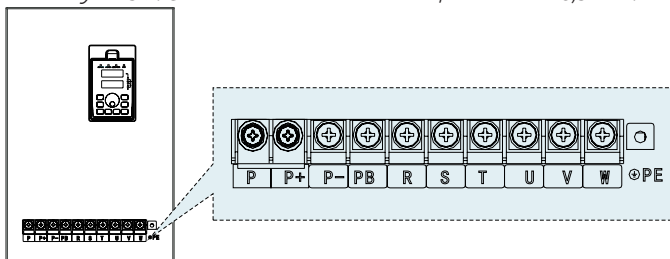
Рисунок 3-10. Схема силовых клемм ПЧ мощностью 22 кВт.
