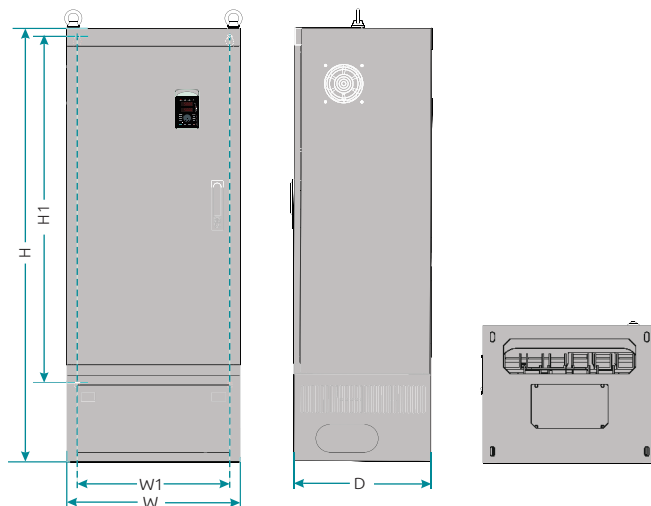
Рисунок 2-10. Установочные размеры ПЧ мощностью 200 — 500 кВт
