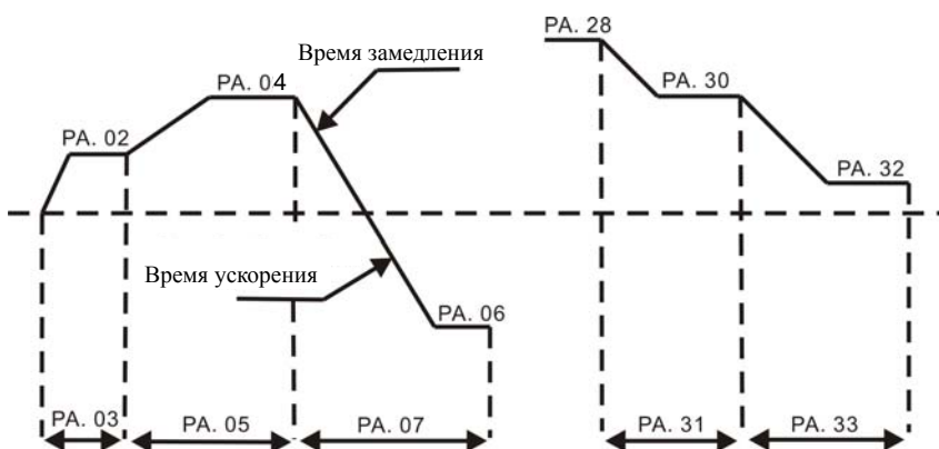
Рис. 6.33 Диаграмма работы под управлением ПЛК
