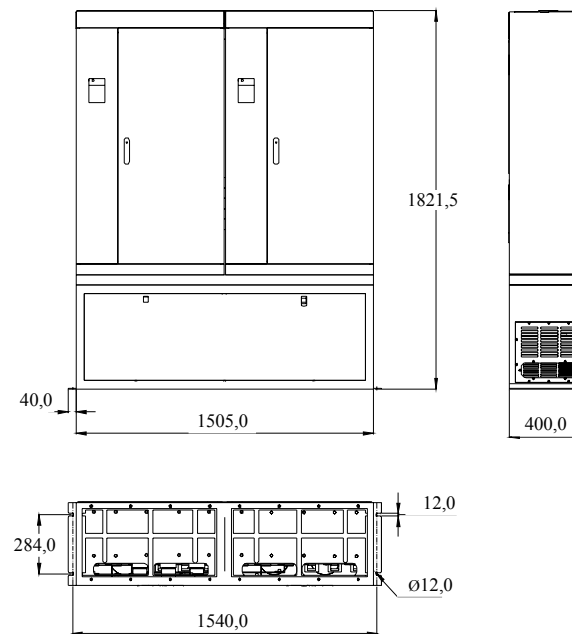
Рис. 1.8 Размеры преобразователей 350 - 630 кВт
