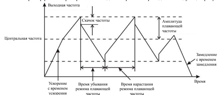
Рис. 6.21 Иллюстрация режима плавающей частоты
