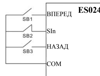
Рис. 6.16 Режим 3-проводного управления 2
