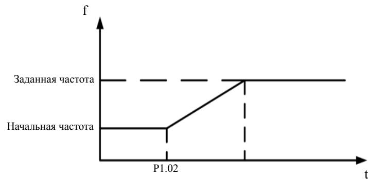
Рис. 6.4 Диаграмма запуска
