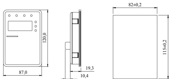
Рис. 3.5 Габаритные и установочные размеры большого пульта
