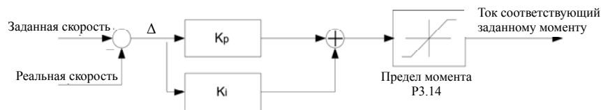
Рис. 6.8 Структура АРС
