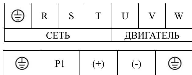
Рис. 4.6 Расположение силовых клемм преобразователей мощностью от 350 до 630 кВт
