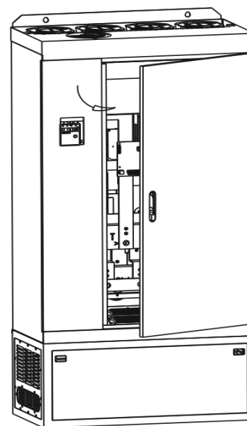
Рис. 3.8 Открывание дверцы преобразователя шкафного исполнения
