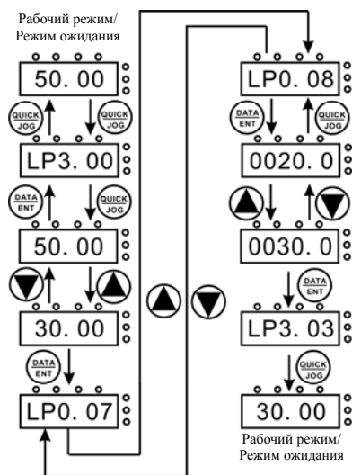
Рис. 5.3 Работа с меню быстрого доступа
