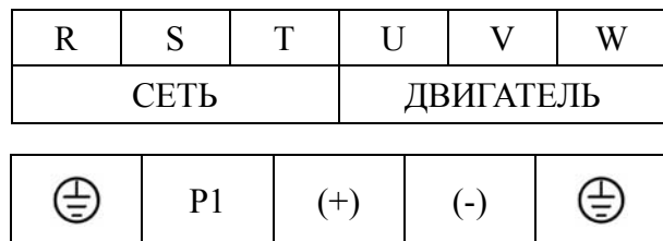
Рис. 4.5 Расположение силовых клемм преобразователей мощностью от 132 до 315 кВт
