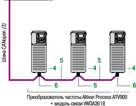
Пример подключения преобразователей частоты к шине CANopen при помощи разъемов типа SUB-D
