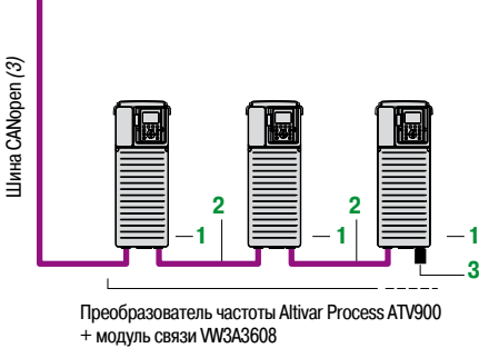
Оптимальное решение - подключение преобразователей частоты «шлейфом» на шину CANopen
