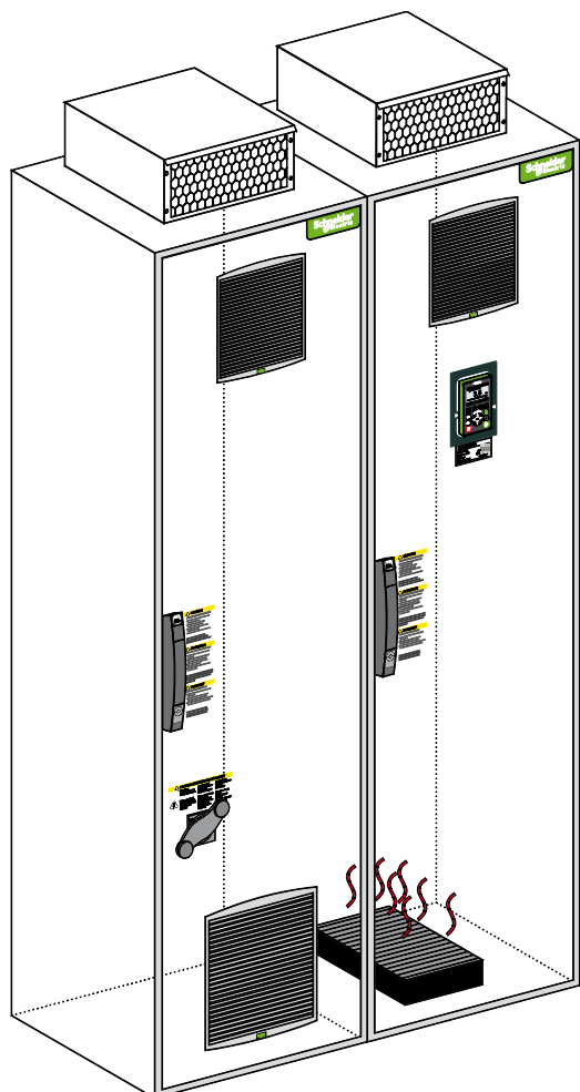
Обогрев шкафа
