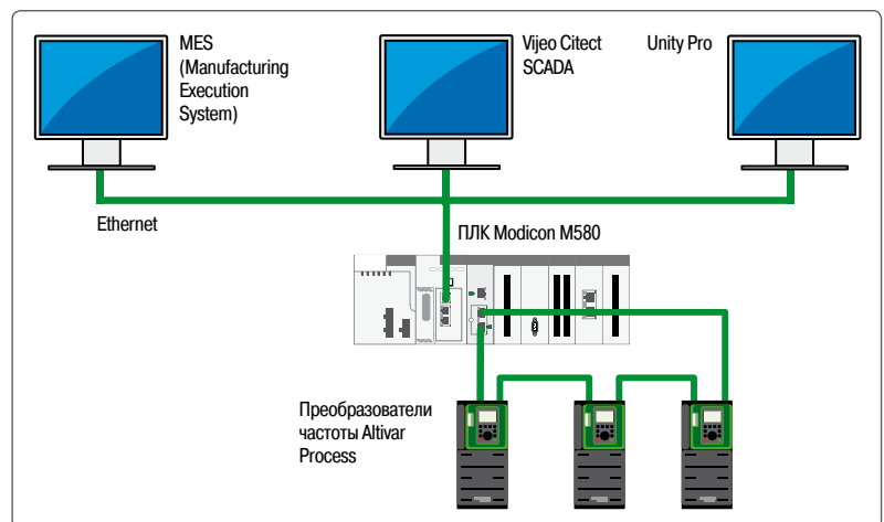
Пример использования в системе автоматизации, построенной на платформе Modicon M580
