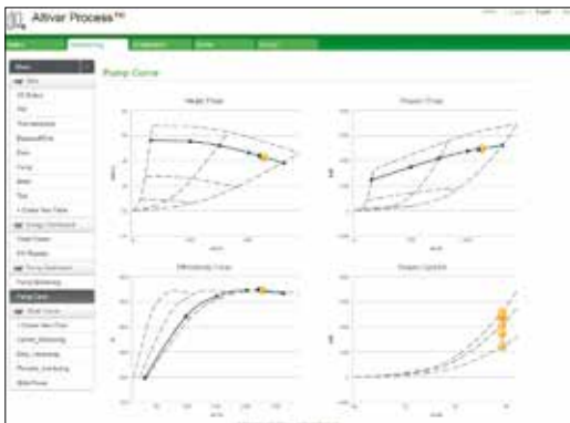
Характеристики насосного агрегата
