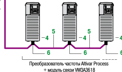
Шина CANopen (3)
