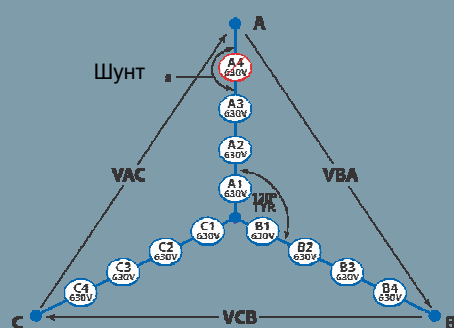
Эквивалентная цепь с 4 ячейками привода Perfect Harmony 3-го поколения с неисправной ячейкой A4
