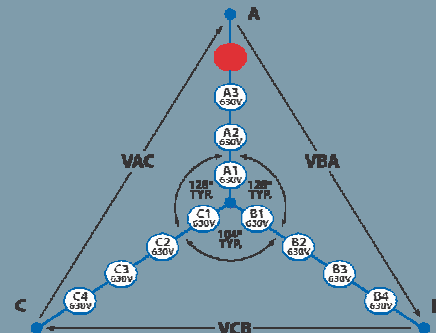
Эквивалентная цепь с 4 ячейками 3-го поколения привода Perfect Harmony с неисправной ячейкой A4
