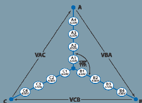
Эквивалентная цепь с 4 ячейками привода Perfect Harmony 3-го поколения при нормальной работе всех рабочих ячеек
