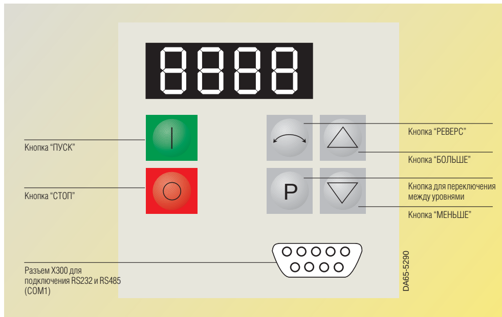
Рис. 2/5 Панель управления и параметризации PMU
