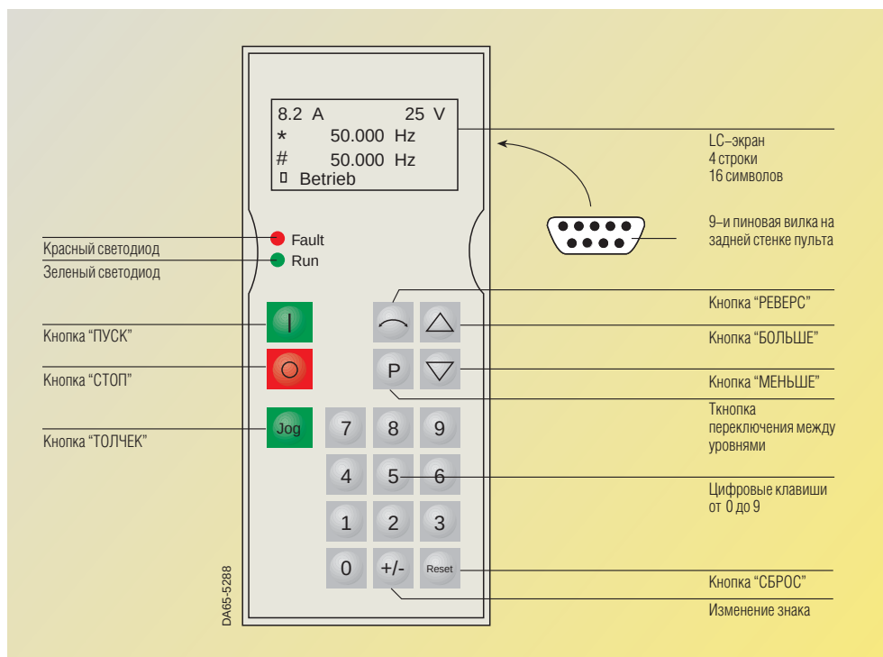
Рис. 2/7 Пульт OP1S
