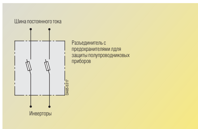
Рис. 6/36 Электромеханическое подключение
