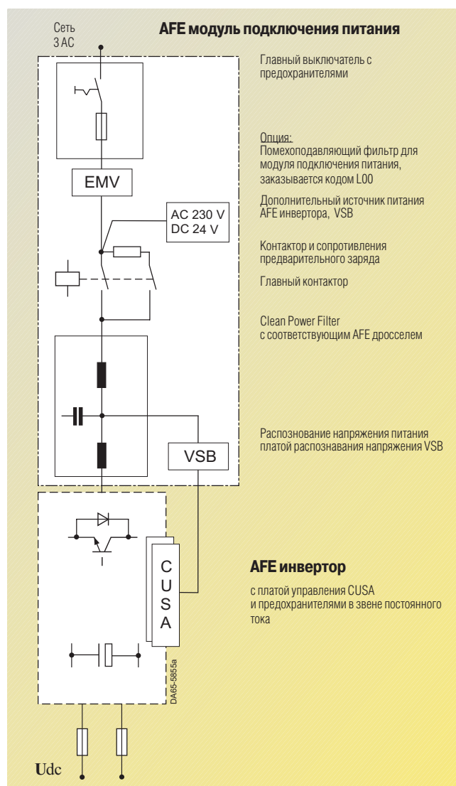
Рис. 3/4 AFE блок встраиваемого исполнения
