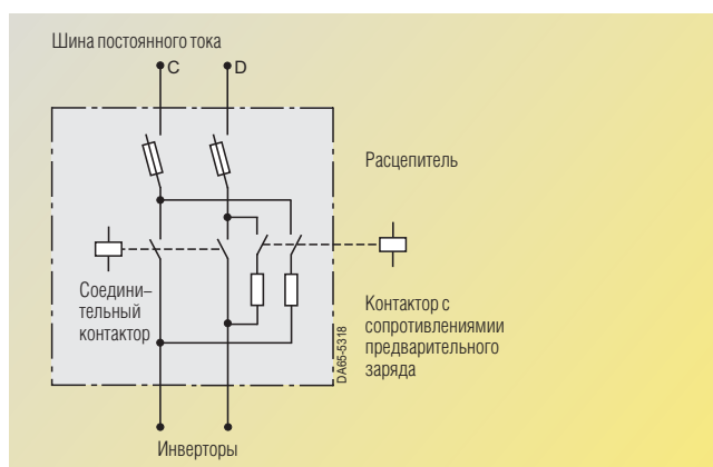
Рис. 6/37 Электрическое подключение
