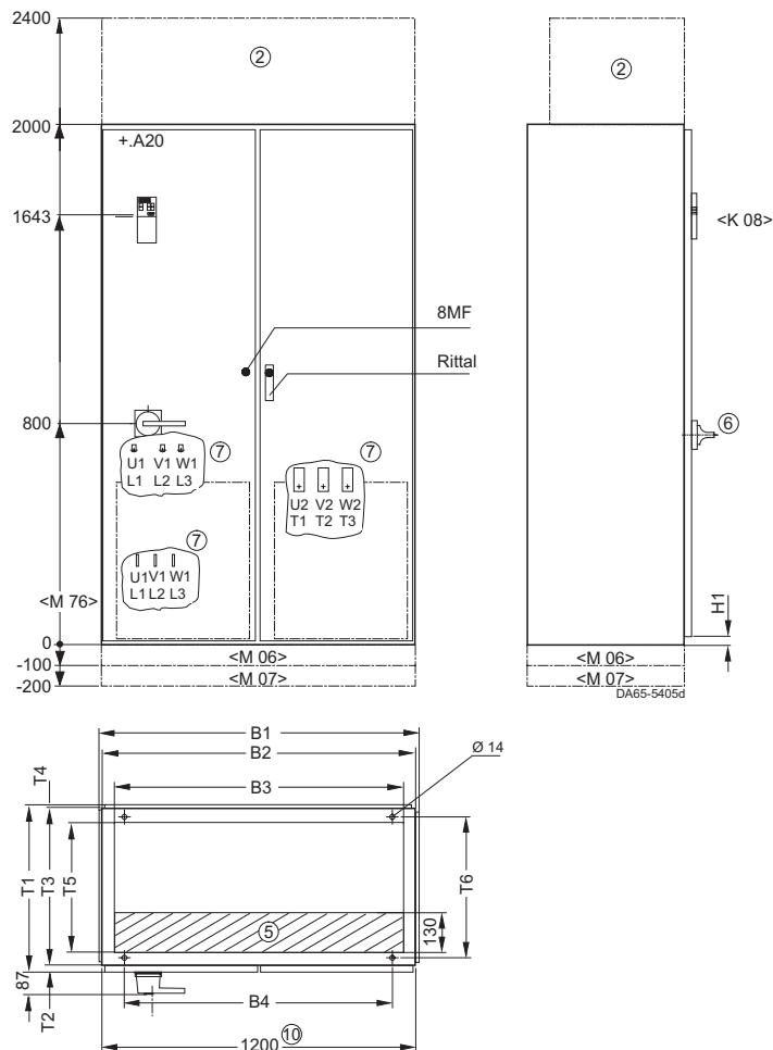
Шкаф Тип B1 B2 B3 B4 T1 T2 T3 T4 T5 T6 H1 8MF 1218 1200 1140 1050 634 25 600 9 466 510 63 Rittal 1202 1199 1112 1075 602 6,5 589 6,5 440 470 25,5
